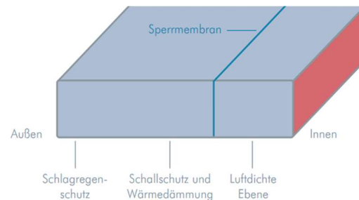
3- Ebenen Funktionsaufbau (schematische Darstellung)
